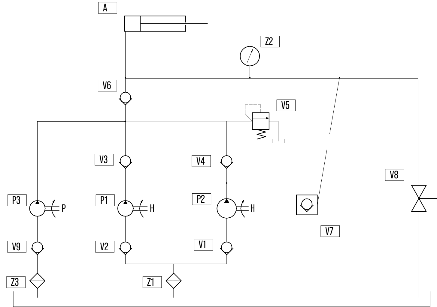
16.1.4 Schema idraulico
